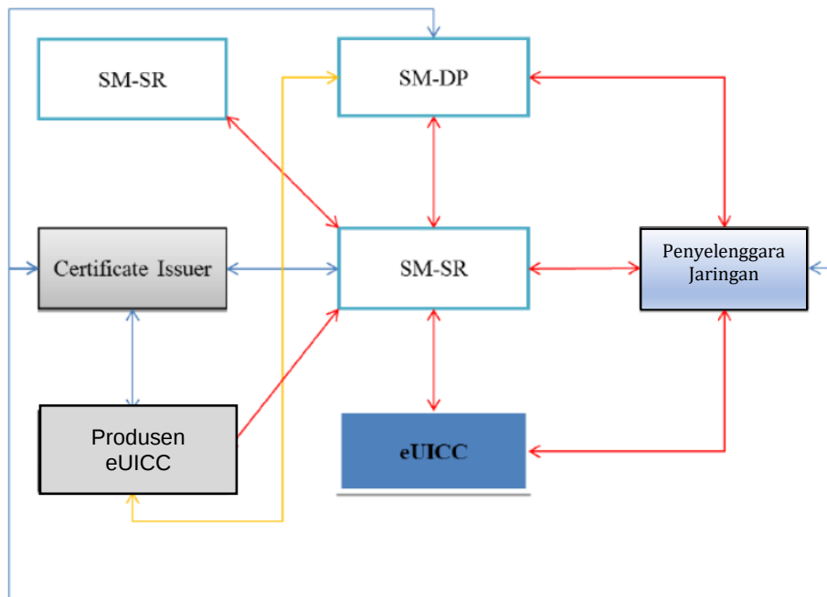
Gambar 3. Arsitektur Provisioning eSIM Jarak Jauh pada Perangkat M2M
